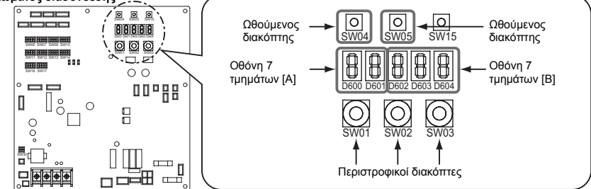
Πλακέτα τυπωμένου κυκλώματος διασύνδεσης
