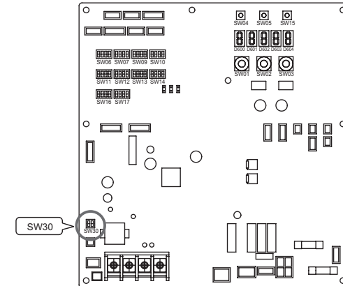
Ηλεκτρονική πλακέτα διασύνδεσης της κύριας μονάδας
