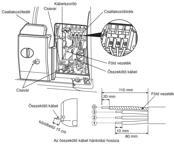
Az összekötő kábel hántolási hossza
