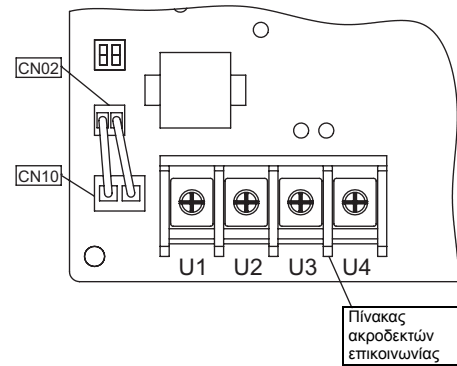
[U1, U2] και [U3, U4] συνδεδεμένα
