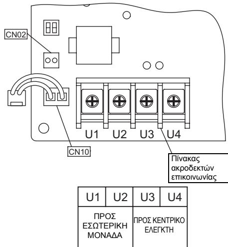
[U1, U2] και [U3, U4] μη συνδεδεμένα
